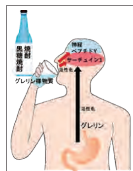
▲ 黒糖焼酎・芋焼酎に含まれるグレリン様物質の作用
