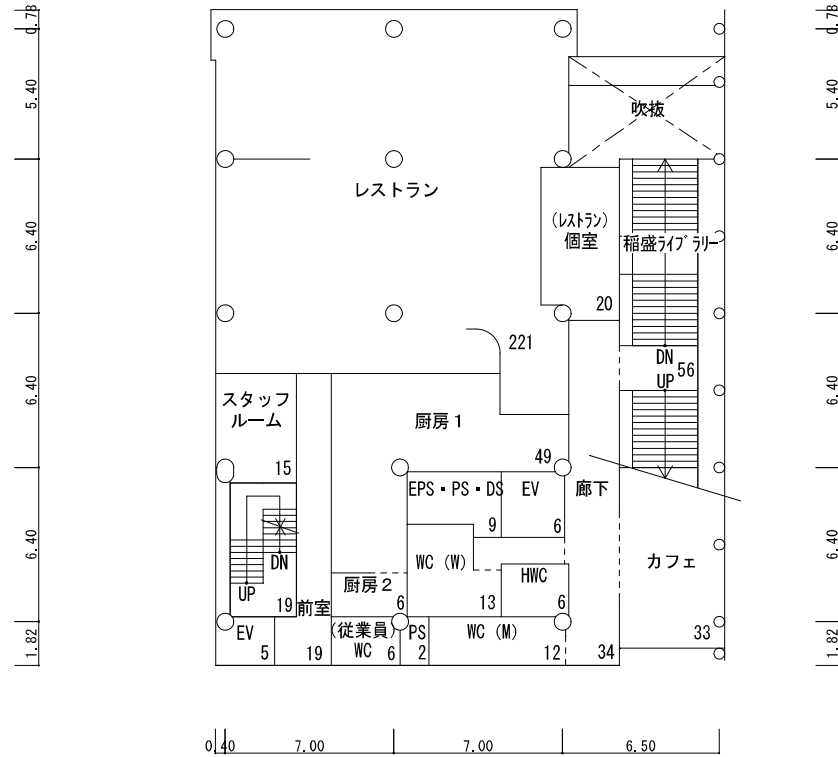
(390) 2 階 平 面 図 S=1/300 531m 2
