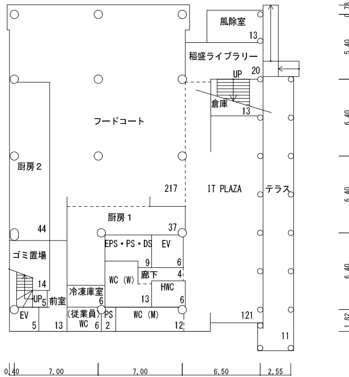
(390) 1 階 平 面 図 S=1/300 577m 2
