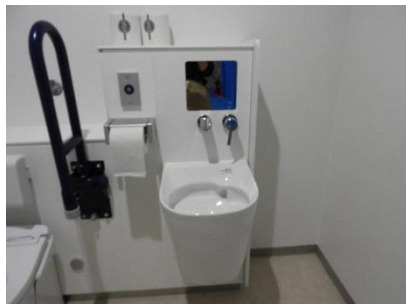
1 階みんなのトイレ個室オストメイト
